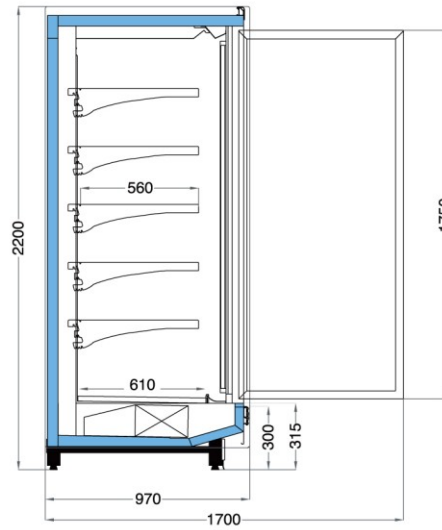
AMATIS LT 2200
