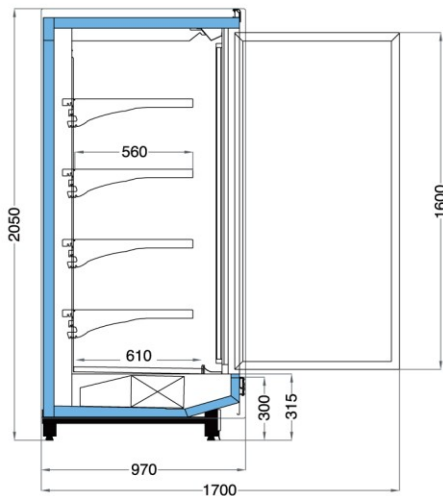
AMATIS LT 2050
